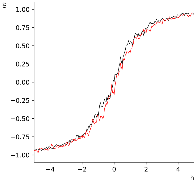
Hystérésis de l'aimantation réseau de taille L=32 - h=5 à T=5
