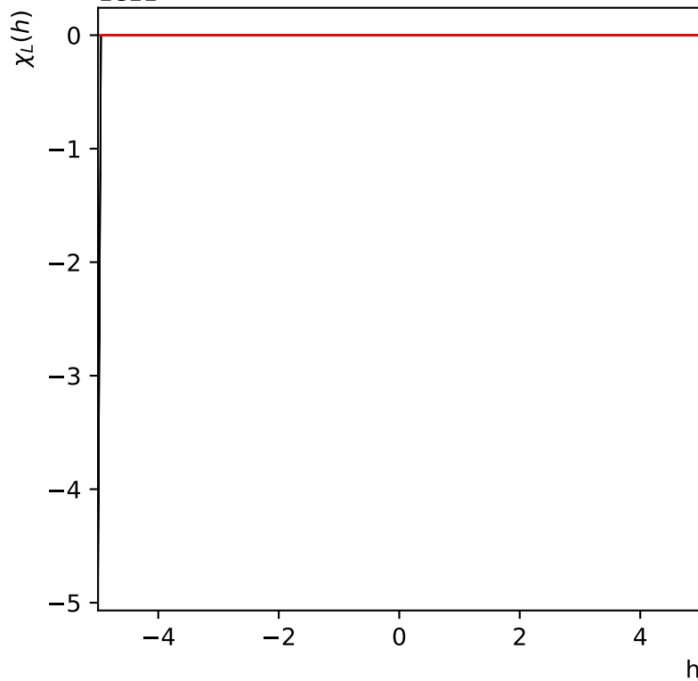
\chi_L(h) réseau de taille L=32 à T=5
